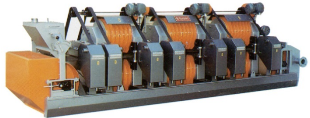
Séparateurs à bande croisée Cross belt separators
